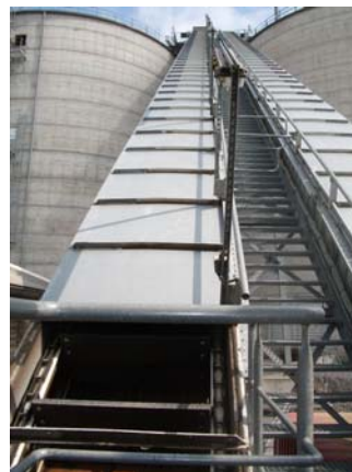
Biomassekraftwerk Förderkettenband mit Mitnehmern aus obo-Festholz®
